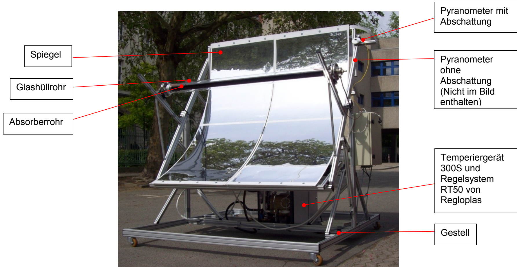
Bild 1: Aufbau des Parabolrinnen-Versuchsstands
