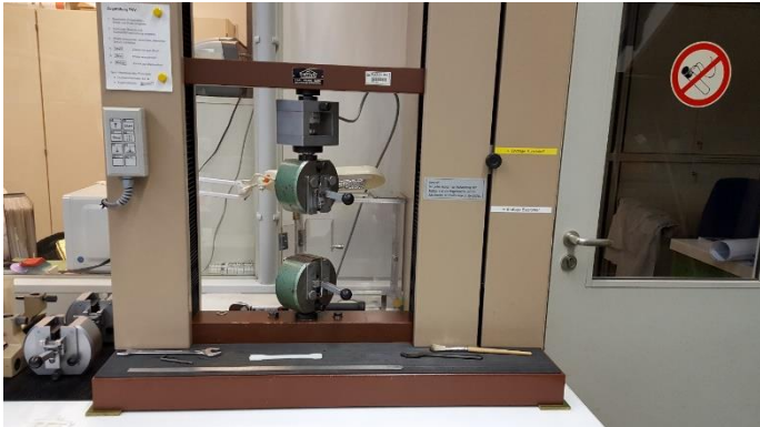
Frank 818 Zugprüfmaschine für Spritzgießteile, Rundprofile und FKV
