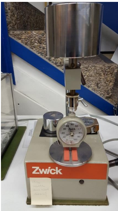
Zwick 7206 Shore Härteprüfung
